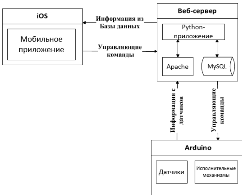
Рис. 1. Архитектура решения.
