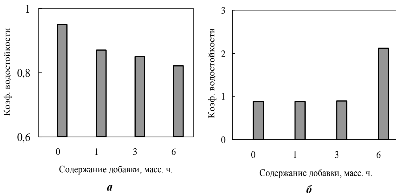
Рис. 1. Зависимость изменения коэффициента водостойкости ненаполненных (а) и наполненных (б) эпоксидных композитов после 9 часов выдерживания образцов в воде при t = 80\text{ }^{\circ}\text{C} от содержания биоцидной добавки.
