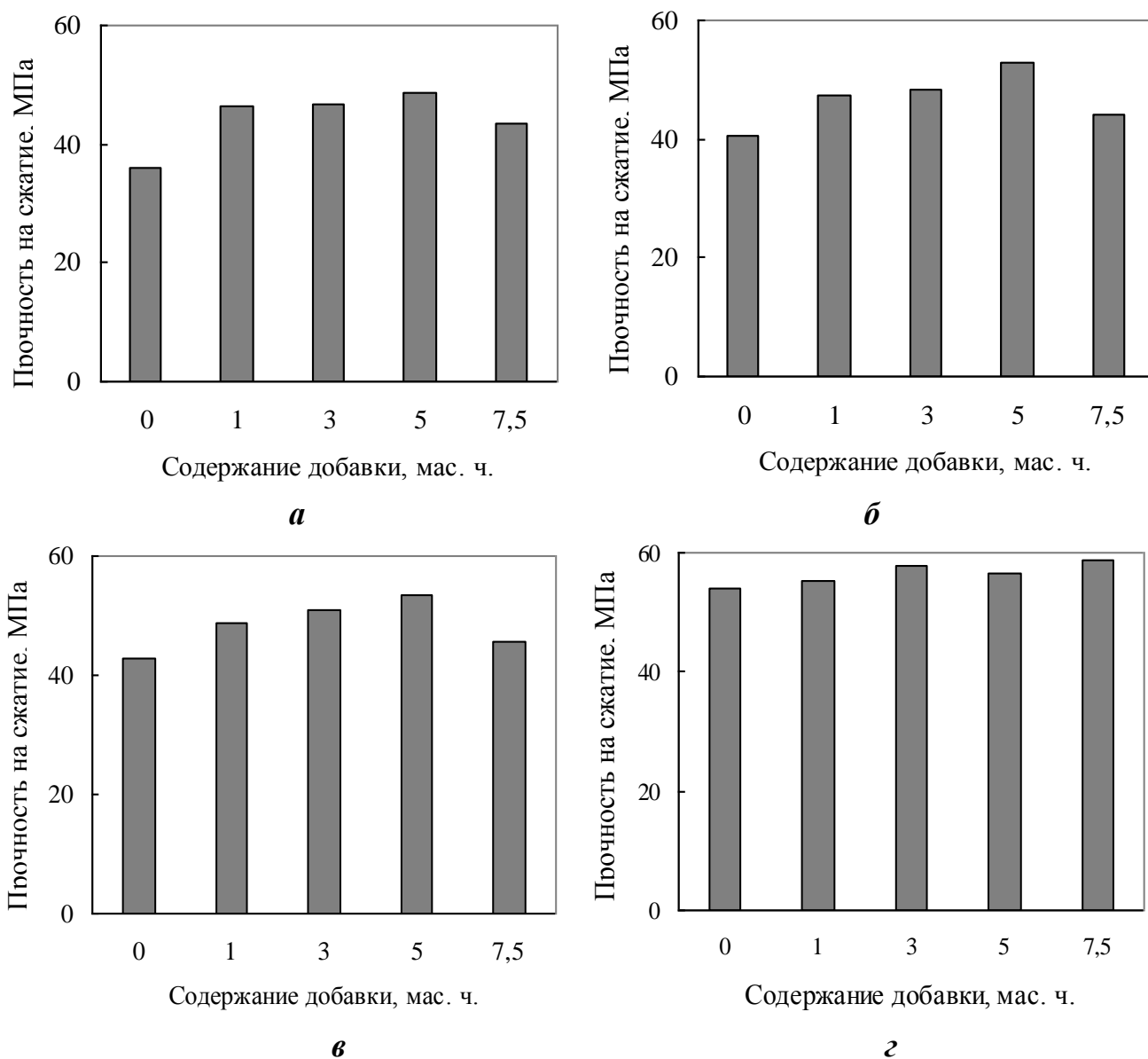
Рис. 4. Зависимость изменения прочности на сжатие композитов на основе портландцемента М500 Д0 от условий твердения и содержания добавки «Тэфлекс Индустриальный»: а – композиты, твердевшие в нормальных условиях в течение 7 суток; б – то же 14 суток, в – то же 14 суток, г – композиты, отвержденные в условиях термовлажностной обработки.
