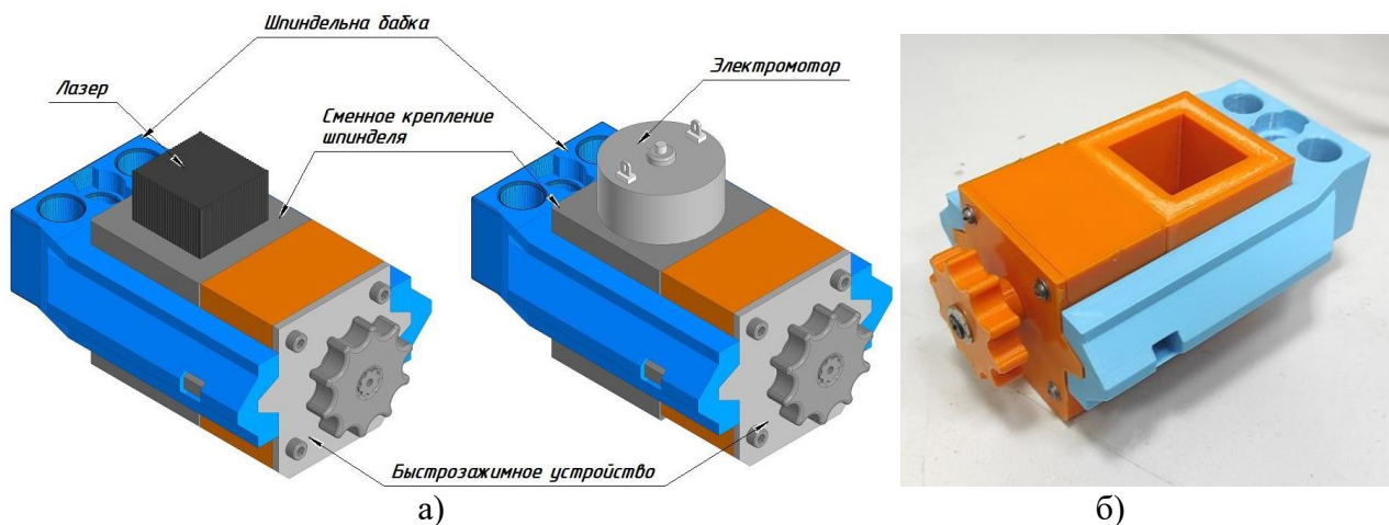
Рис. 4. Быстрозажимное устройство для шпиндельной бабки в виде 3D-модели (а) и в реальном исполнении (б).
