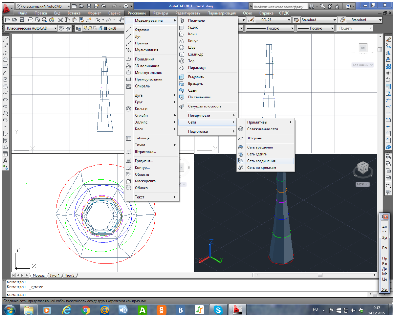
Рис. 9. Трёхмерная модель антенно-мачтового сооружения.
